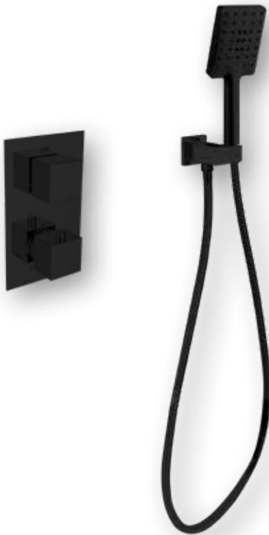
53.8001N Regadera London black → 275 ↑ 105 ↗ 532 mm London desviador → 120 ↑ 200 ↗ 55 mm
